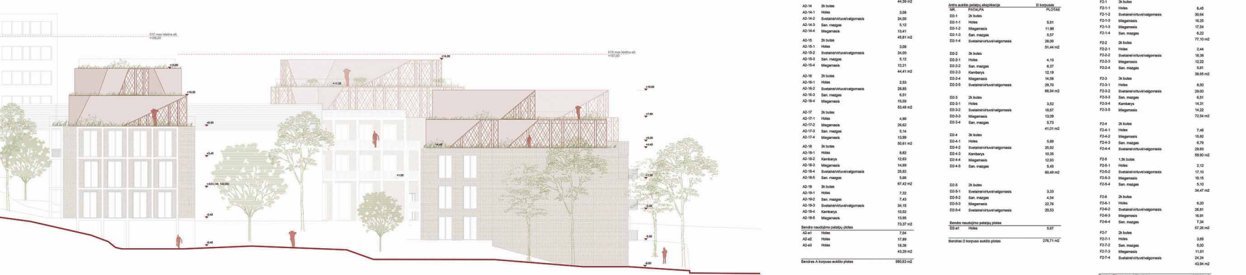
KIEMO KORPUSŲ IŠKLOTINĖ M 1:200
