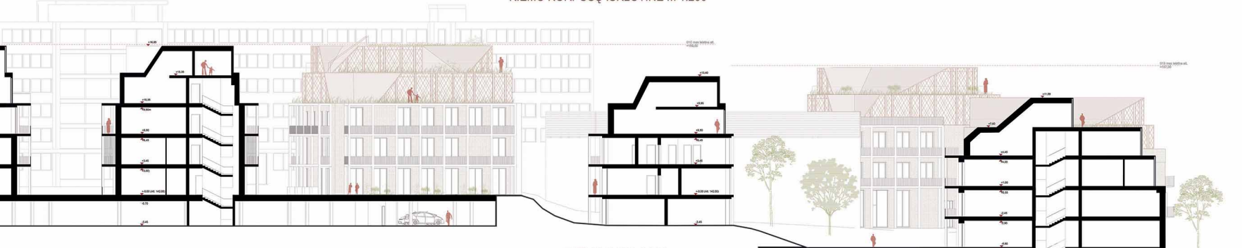
PJŪVIS 2-2 M 1:200
