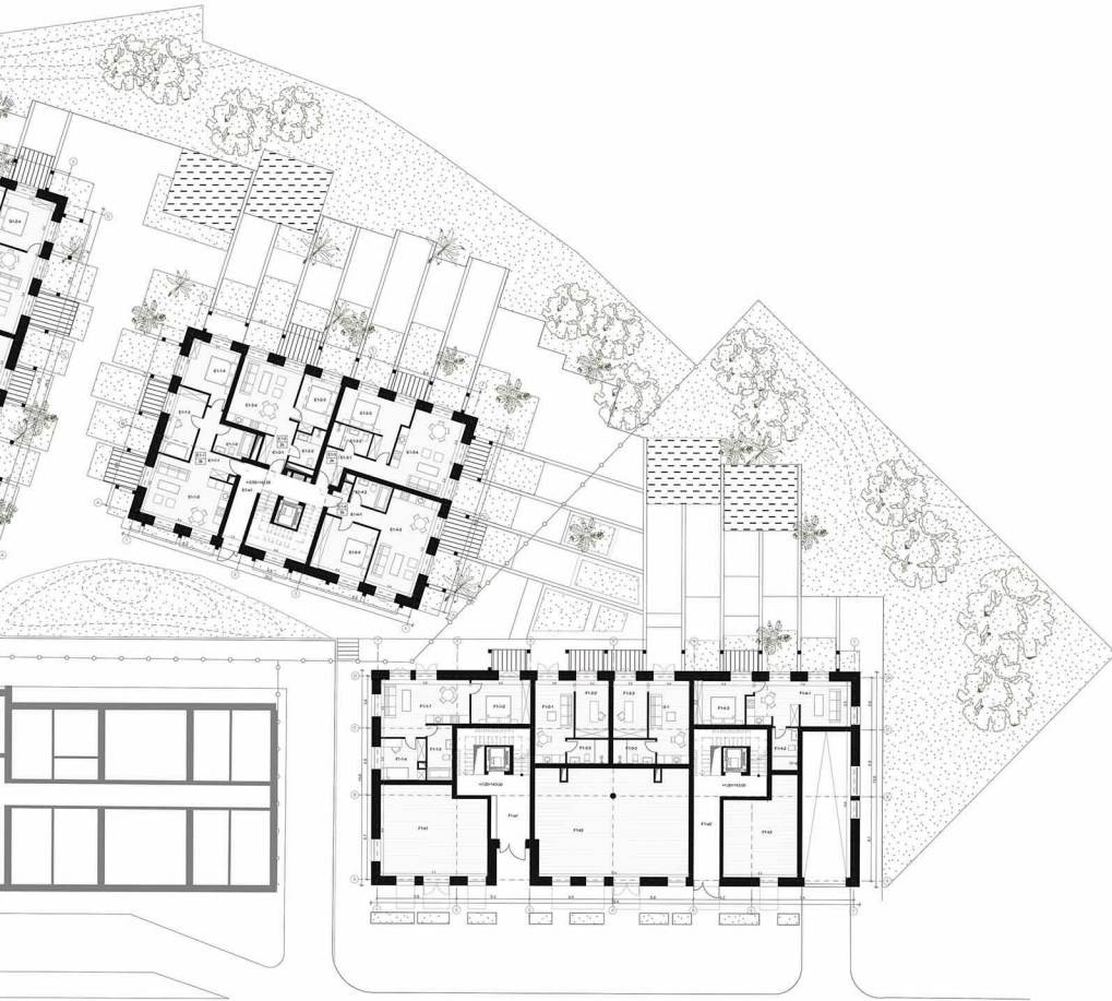
PIRMO AUKŠTO PLANAS M 1:200
