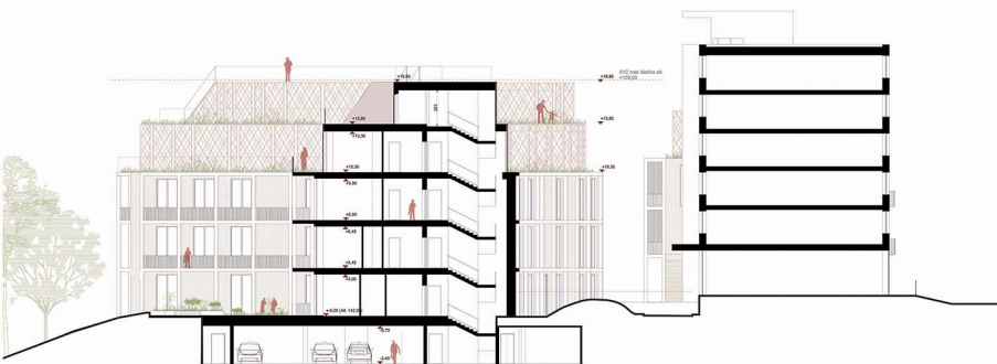
PJÜVIS 1-1 M 1:200
