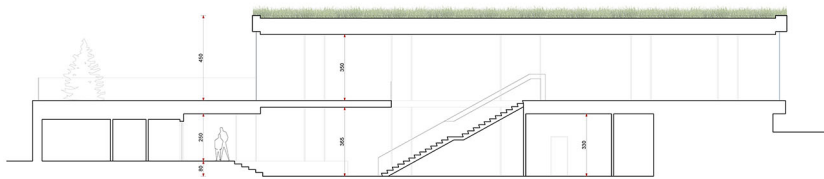
PJŪVIS A
