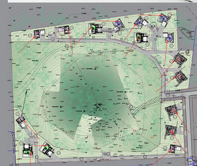
SAULĖS SPINDULIŲ PATEKIMO SCHEMA
